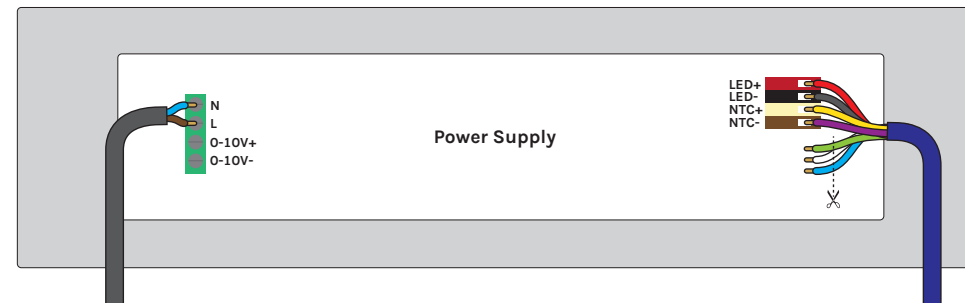
Conexiones a la fuente de alimentación de la lámpara subacuática MONO (sin regulador)
