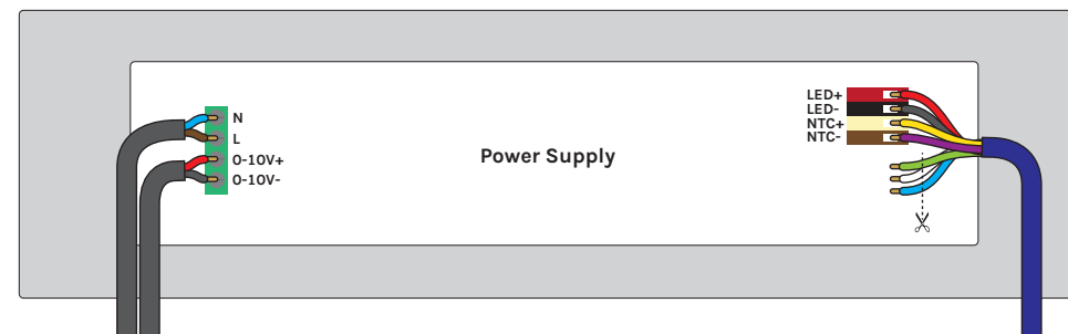
Conexiones a la fuente de alimentación de la luz subacuática MONO (con regulador de intensidad de 0 a 10 V CC)
