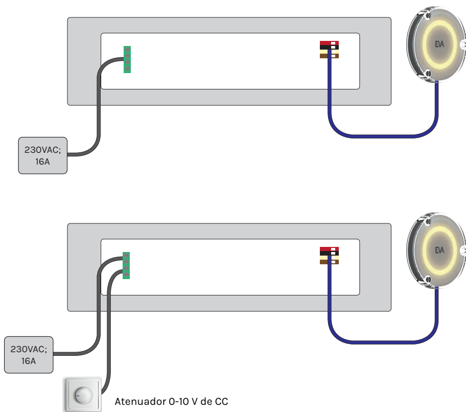
Vista general - Combinación de lámparas subacuáticas MONO SubAqua LED y fuentes de alimentación
